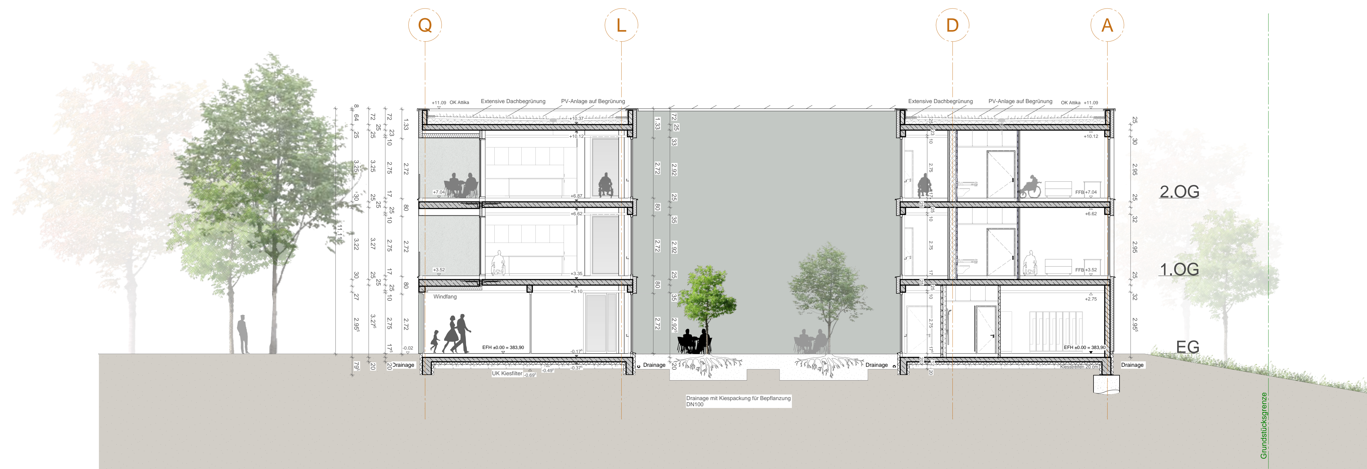
SCHNITT B-B
