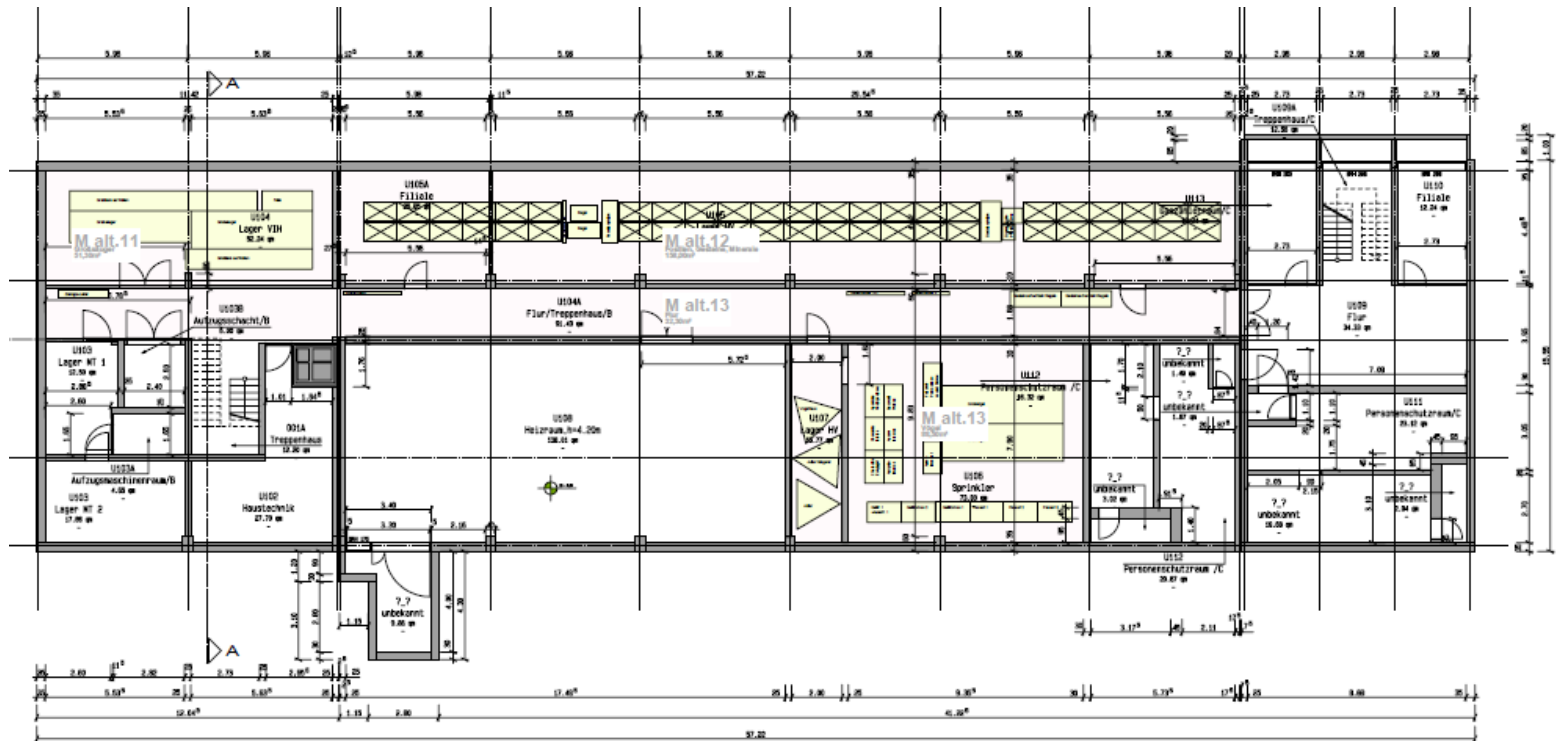
Untergeschoss
