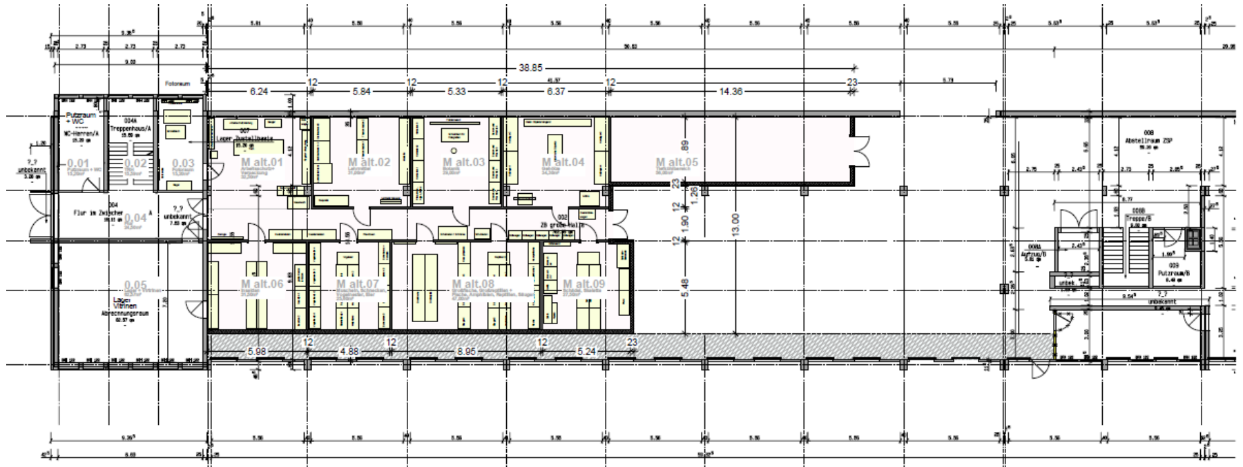
Erdgeschoss
